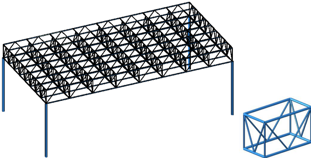
Рис. 1. Моделі сталевій плити покриття, яка досліджується: модель 1 з базовим формоутворюючим елементом 1-го типу-а; модель 2 з базовим формоутворюючим елементом 2-го типу -б
